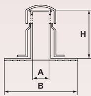
Tipo Semplice Simple wall roof vent
