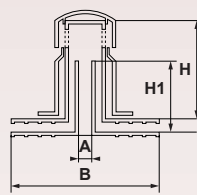
Tipo Doppio Double wall roof vent
